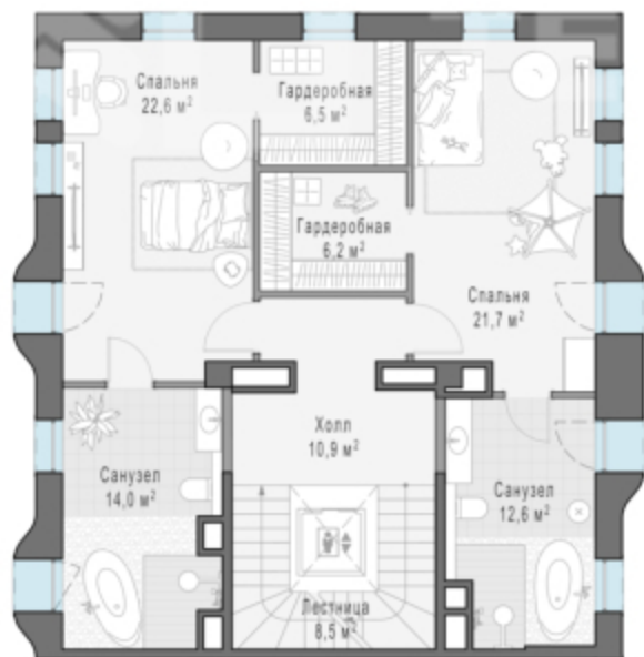
3 этаж
